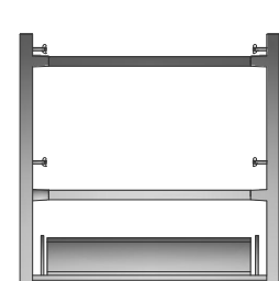
BARANDA LATERAL DE TERMINO STD 125 Y 100 PESO : 13.10 Kg
